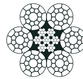
6x19 Seal + IWRC
