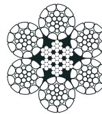
6x26 WS + IWRC
